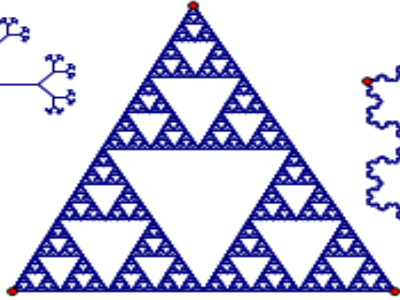
Sierpinski Gasket
